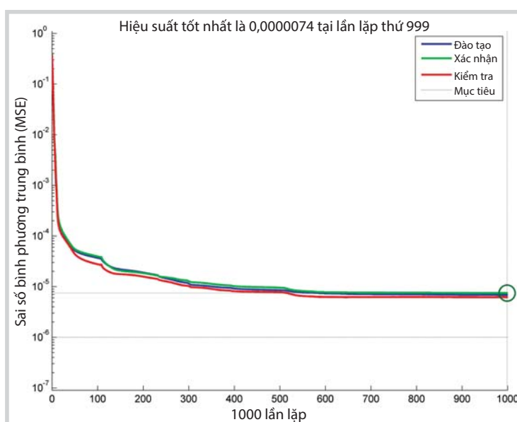
Hình 3. Đồ thị biểu diễn hiệu suất của mạng neural nhân tạo 2-6-5-1
